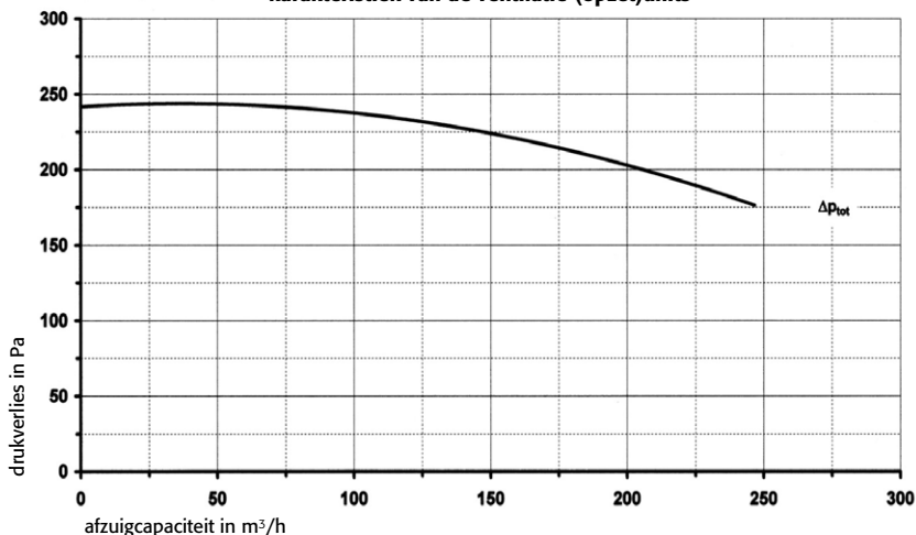
Ventilatie-unit voor onderbouwkasten, voor bevestiging op de muur, met flowbewaking Bestelnr. 14-1025 ■
